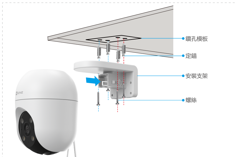
圖 1 天花板安裝
