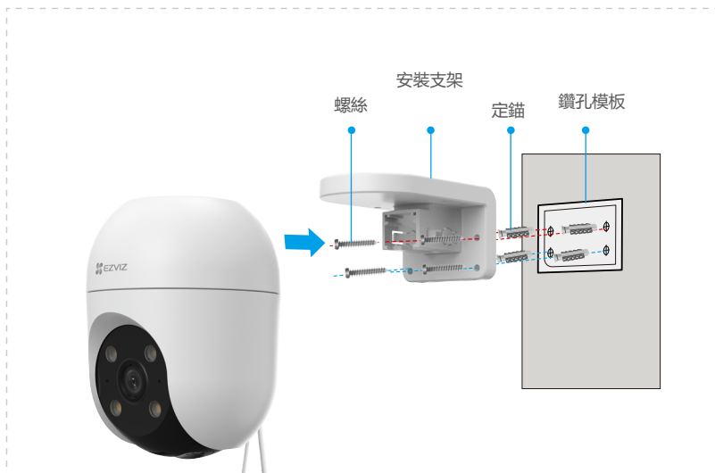
圖 2 壁掛式安裝
